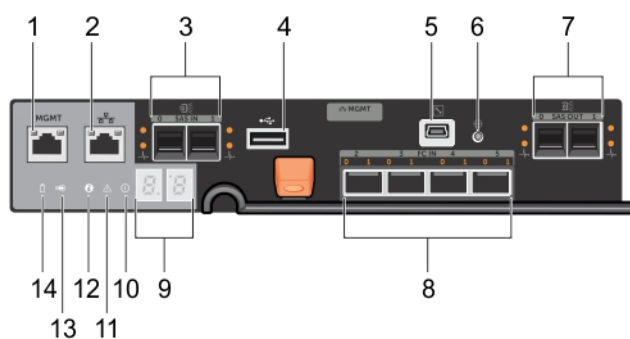
図 8. MD3860f ファイバチャネル RAID コントローラモジュールの機能とインジケータ
