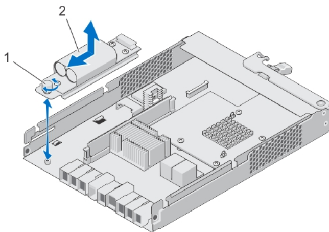
図 25. RAID コントローラモジュールバックアップバッテリーユニットの取り外しおよび取り付け
